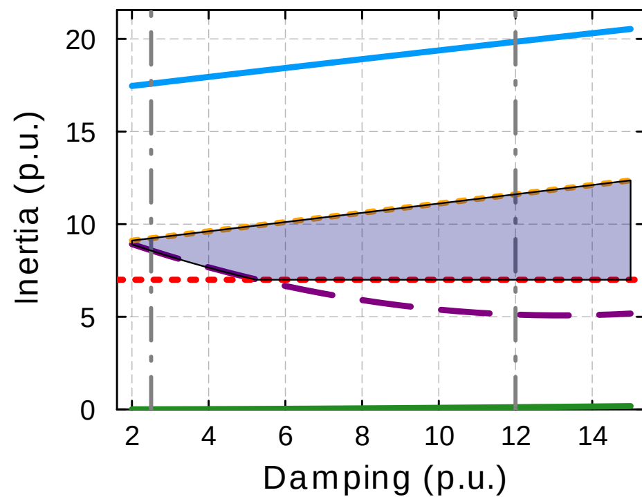
(d) Droop = 0.028
